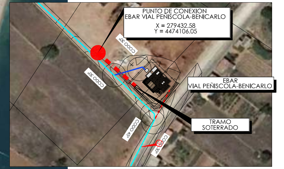
PLANTA ESCALA 1/1000
