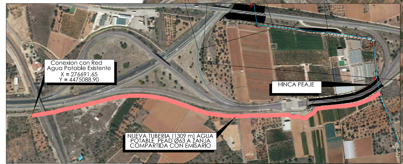
PLANTA ESCALA 1/4000
